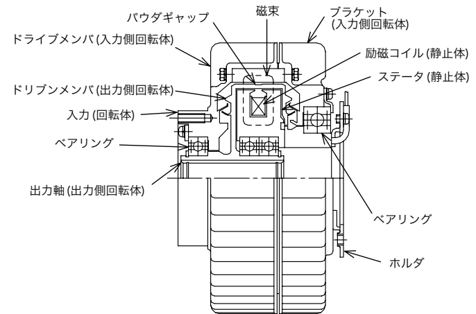
図1 ZA-AN 1 形パウダクラッチ構造図(代表例)
