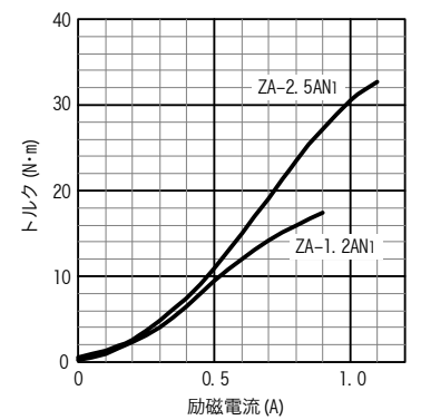
図2 励磁電流対トルク特性(代表例)
