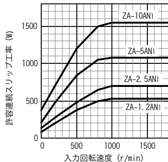
図3 許容連続スリップ工率特性
