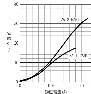
図2 励磁電流対トルク特性(代表例)
