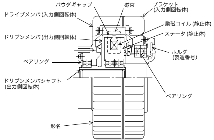
図1 ZA-AN形パウダクラッチ構造図(代表例)
