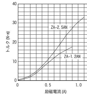
図2 励磁電流対トルク特性(代表例)
