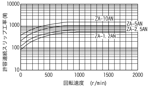
図3 許容連続スリップ工率特性
