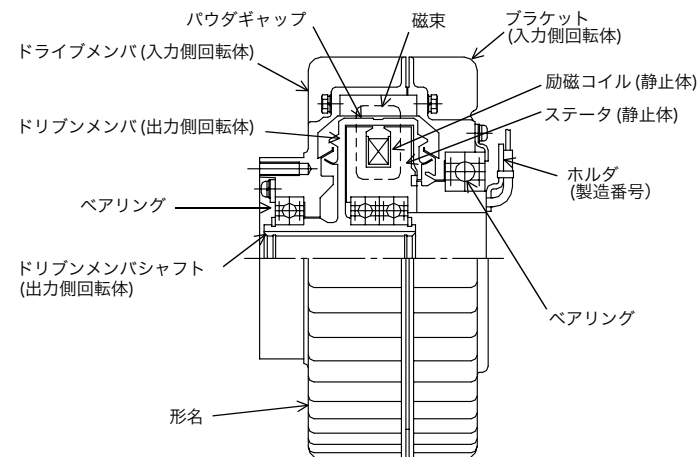
図1 ZA-AN形パウダクラッチ構造図(代表例)
