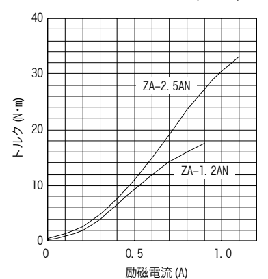
図2 励磁電流対トルク特性(代表例)
