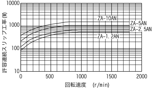
図3 許容連続スリップ工率特性
