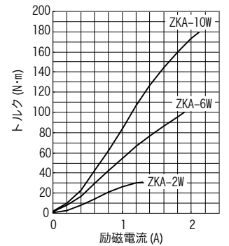
図2 ZKA-W形パワダブレーキ励磁電流対トルク特性(代表例)
