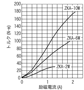
図2 ZKA-W形パウダブレーキ励磁電流対トルク特性(代表例)
