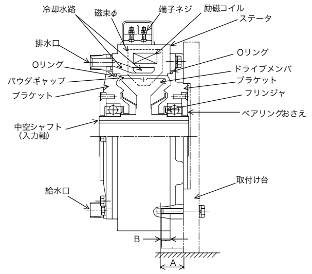
図1 ZKA-W形パウダブレーキ構造図(代表例)
