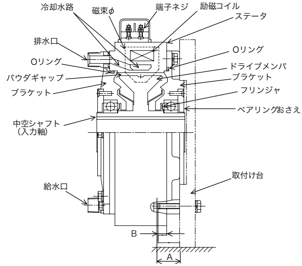
図1 ZKA-W形パワダブレーキ構造図(代表例)
